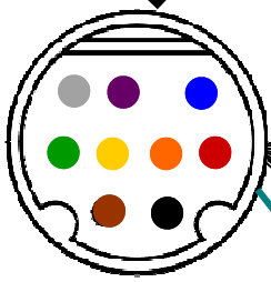
Mini Din 9 Pin Female Connector
